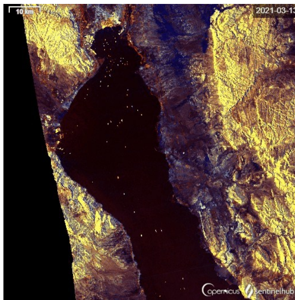
Blokáda Suezského průplavu Sentinel-1
