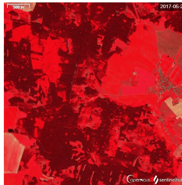
Kůrovcová kalamita v Česku Sentinel-2
